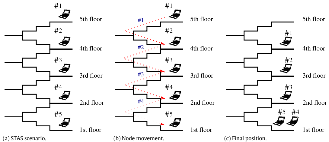
Fig. 1. SHIS scenario.
